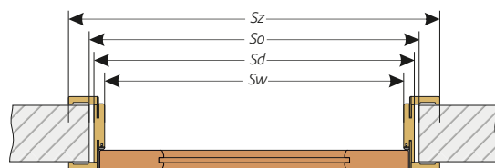
Rozměry obložení bezpodrážkového systému
